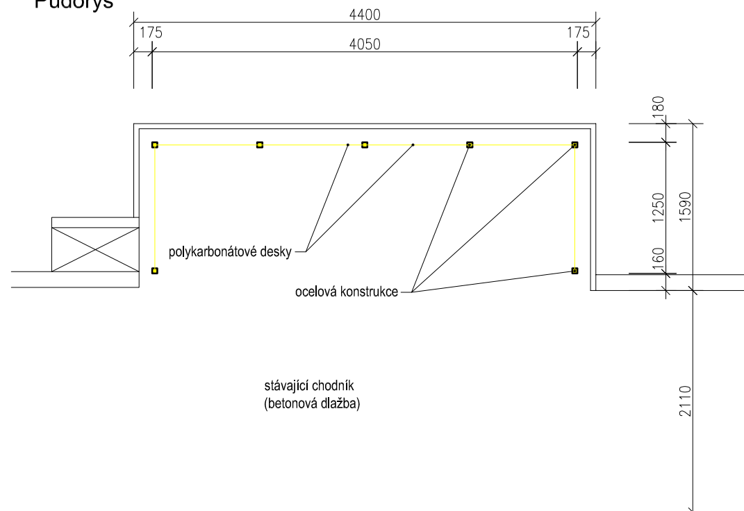
Půdorys
