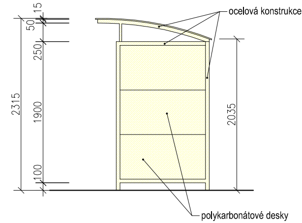
Pohled boční
