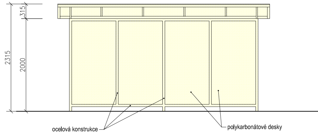
Pohled čelní
