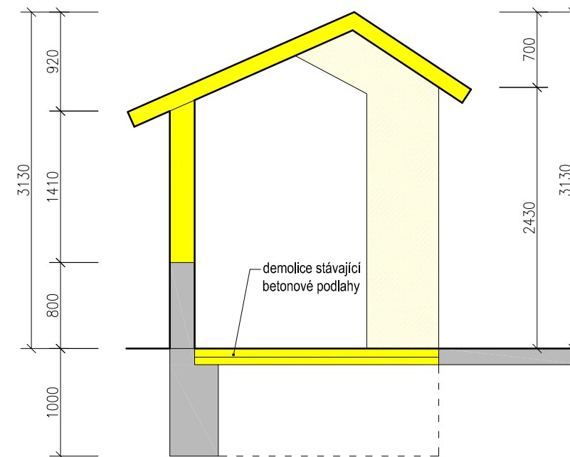
Řez A-A
