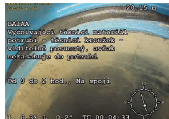
Kamerová prohlídka nového potrubí
